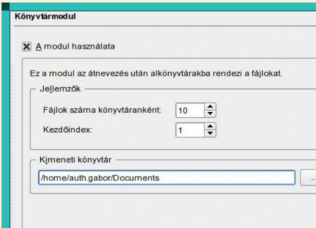
7. ábra Könyvtármodul
