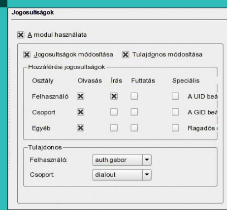
5. ábra Jogosultságok
